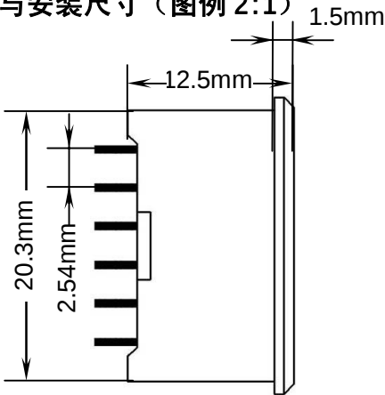
图一：结构与安装尺寸（图例 2:1）
